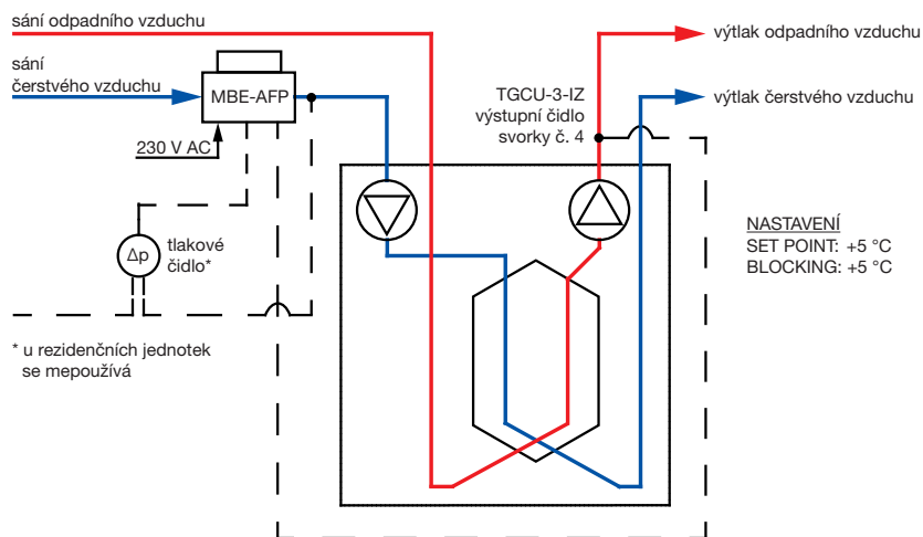
Technologické schéma zapojení elektrického ohřivače v režimu předehřevu (protimrazová ochrana jednotky) za použití externího teplotního NTC čidla.
