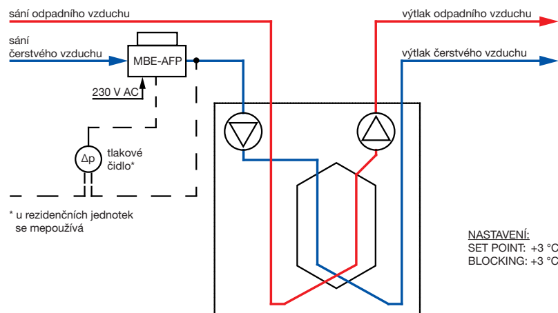
Technologické schéma zapojení elektrického ohřivače v režimu předehřevu (protimrazová ochrana jednotky) bez použití externího teplotního NTC čidla.
