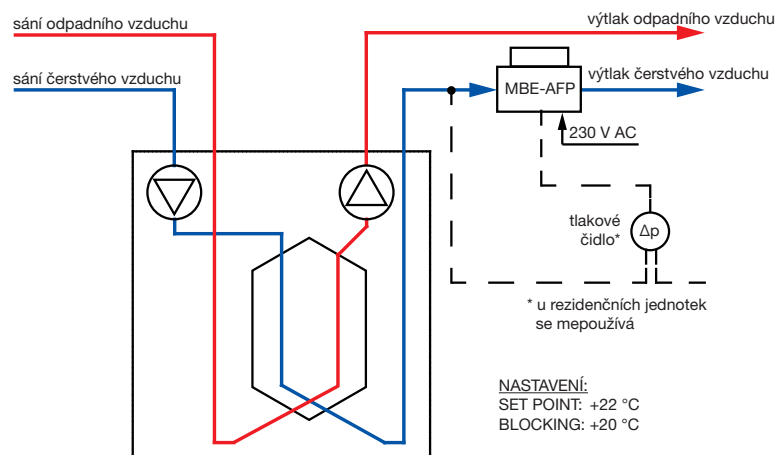
Technologické schéma zapojení elektrického ohřivače v režimu dohřevu přívodního vzduchu (protimrazová ochrana jednotky) bez použití externího teplotního NTC čidla
