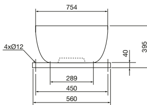
CRVB-N, CRVT-N
