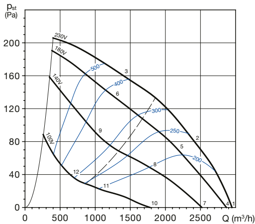
CRHB/6-400 N
