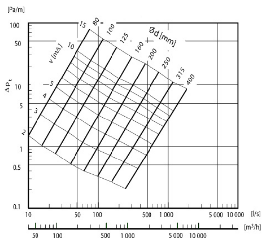
tlakové ztráty tlumičů hluku MAAU
