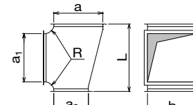
rozbočka šikmá a \times b - a_1 - a_2 - L - R
