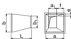
přechod a \times b - a_1 \times b_1 - L
