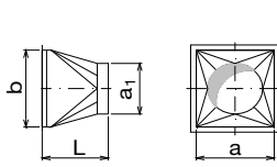
přechod na kruh a \times b - a_1 - L
