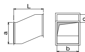
odskok a \times b - o - L
